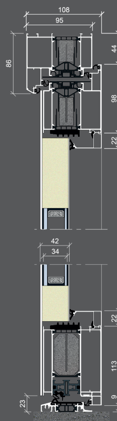
KÖSTER ADVANCE 108 optionale Ausführung mit schrägem Blendrahmen
