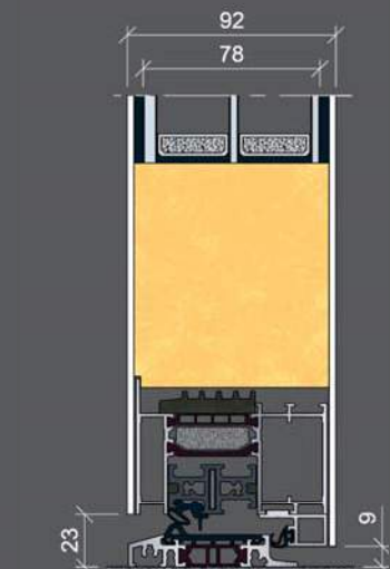
Ausführung mit schrägem Blendrahmen (optional): KÖSTER ADVANCE 108
