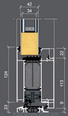
Ausführung mit schrägem Blendrahmen (optional): KÖSTER ADVANCE 108
